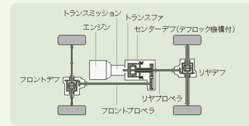
フルタイム4WDシステムイメージ図
