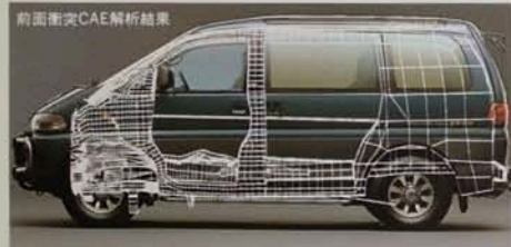
前面衝突CAE解析結果
