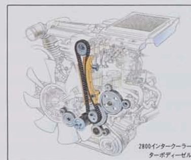
チェーン&ギヤ駆動方式：説明イラスト
