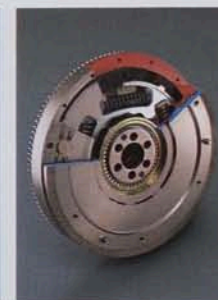
ハイドロフライホイール (2800ディーゼル搭載ワイド車の5M/T) Photo)説明のため、一部をカットしたものです。
