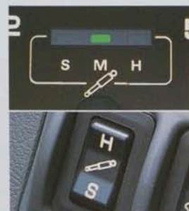
3モード可変ショックアブソーバー (JトップXSとキックアップブルーXEVを除く全車)
